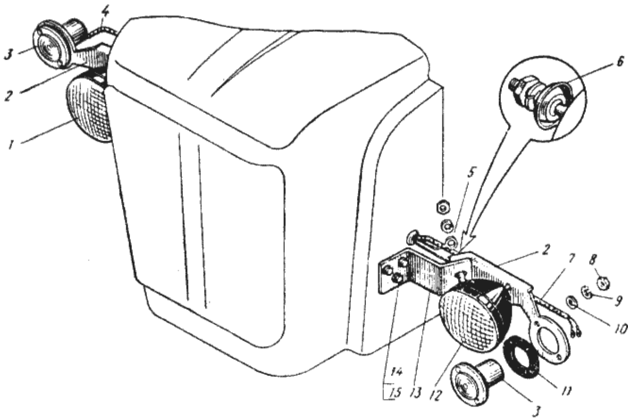
Рис. 50. Установка передних фар
